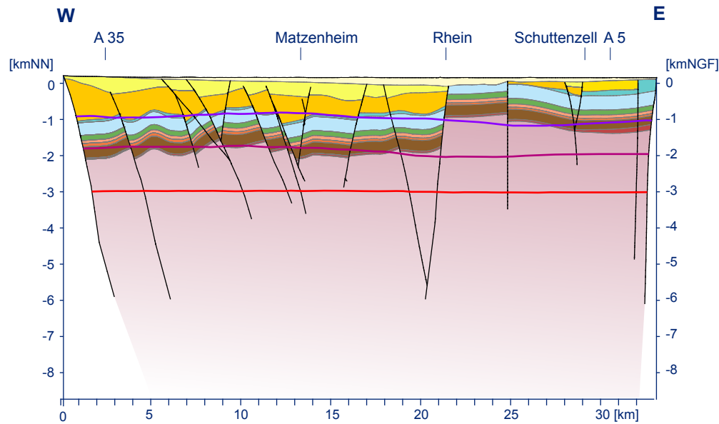
Profil 7
