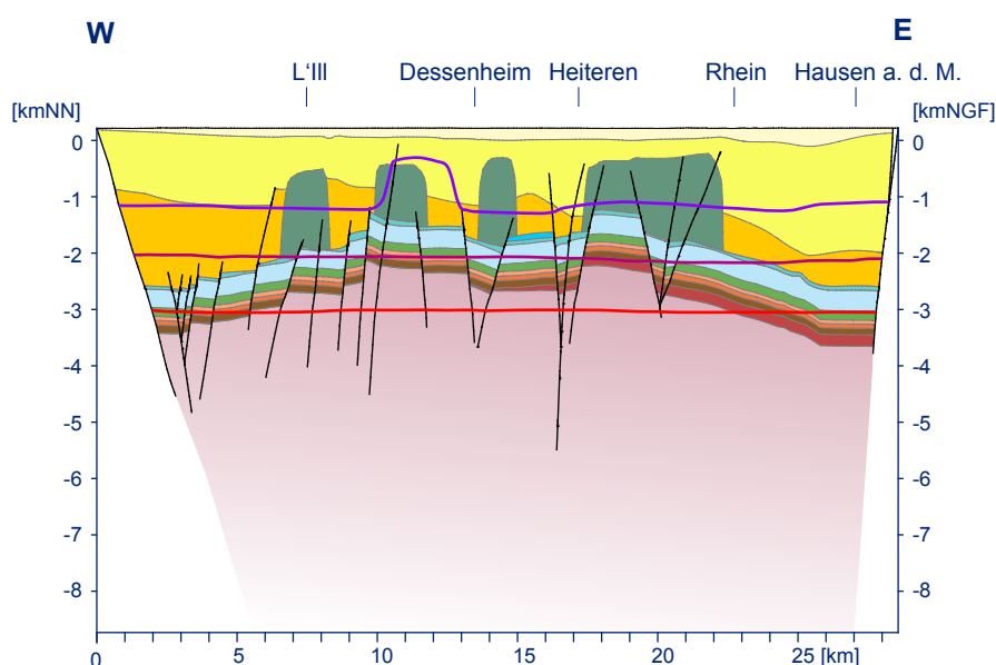
Profil 9
