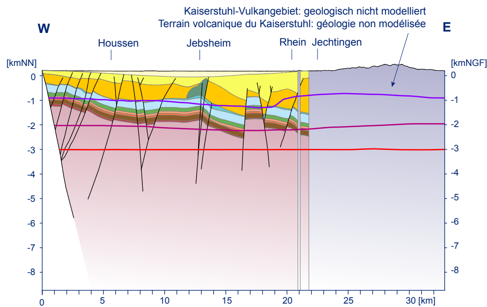
Profil 8
